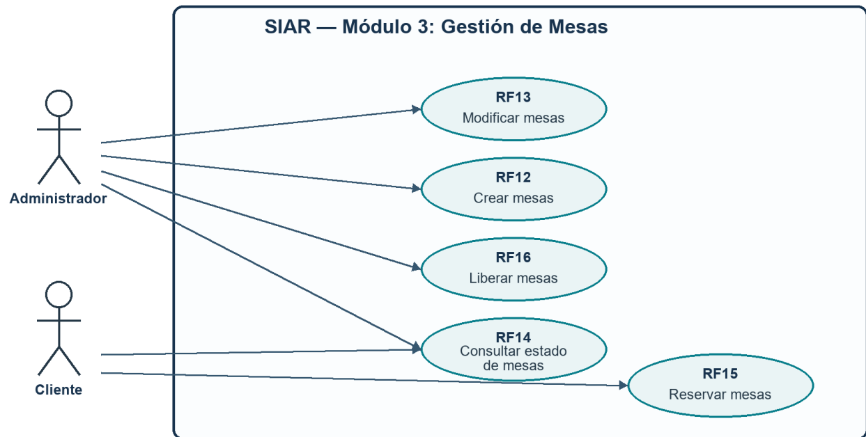
Figura 1. Diagrama de casos de uso del Módulo 3
